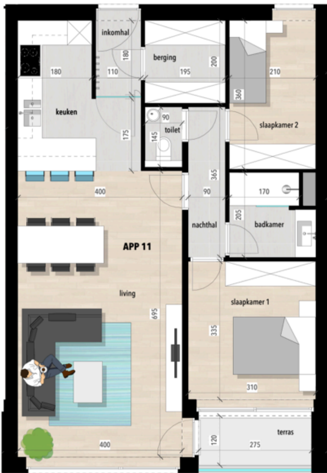
Grondplan 1:75 maten en meubilair zijn indicatief
