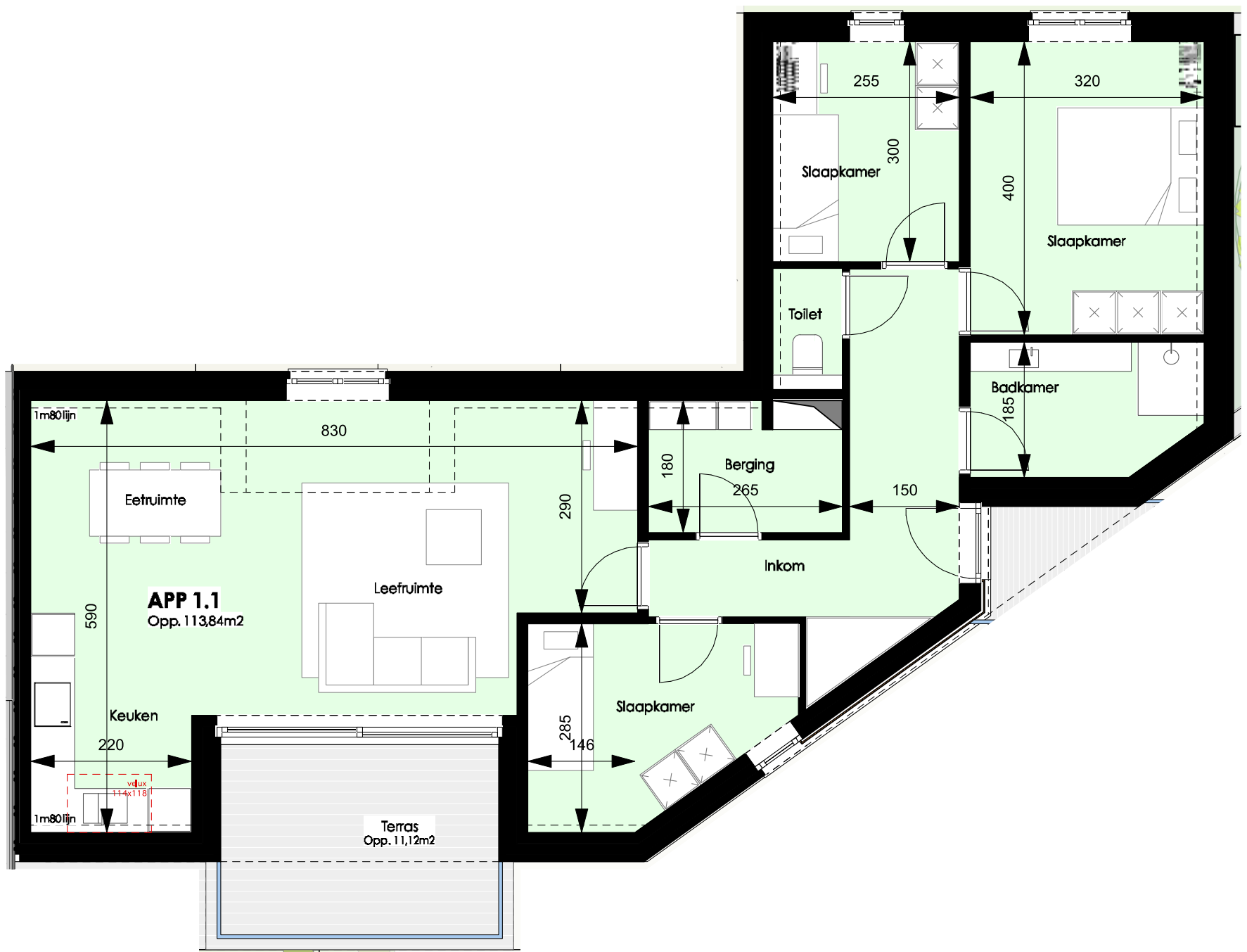
Grondplan
